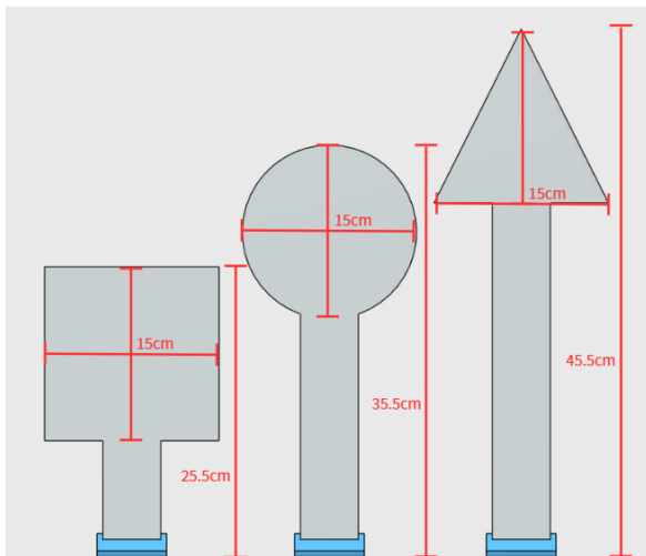
▲標靶參考圖（實際尺寸可能誤差小於 3 mm）
