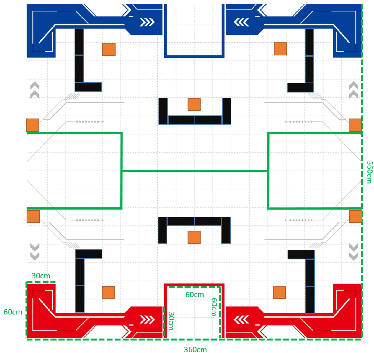
▲標靶爭奪賽競賽場地圖
