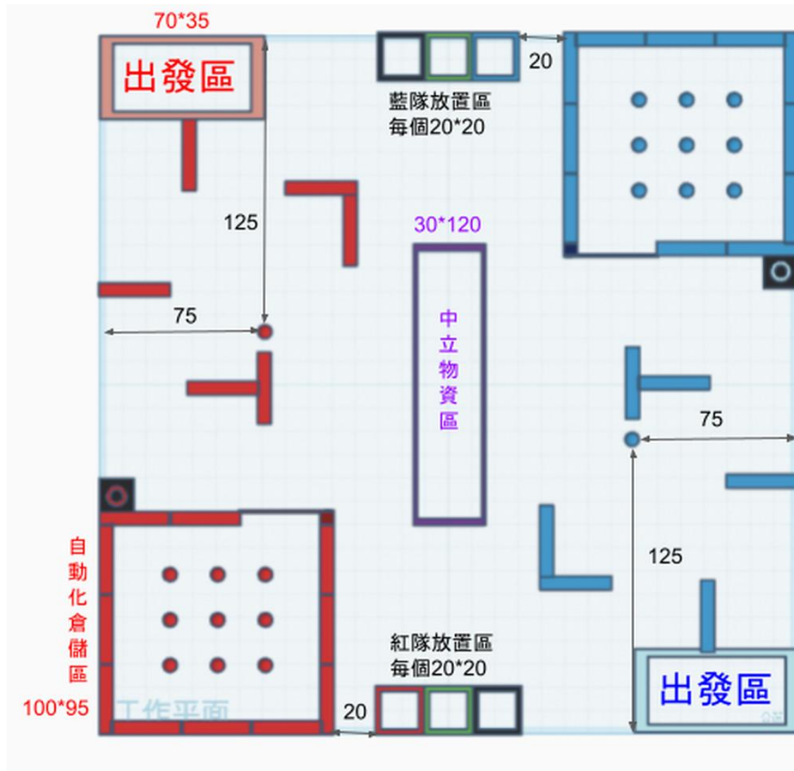
▲物資能源爭霸戰競賽場地俯視圖
